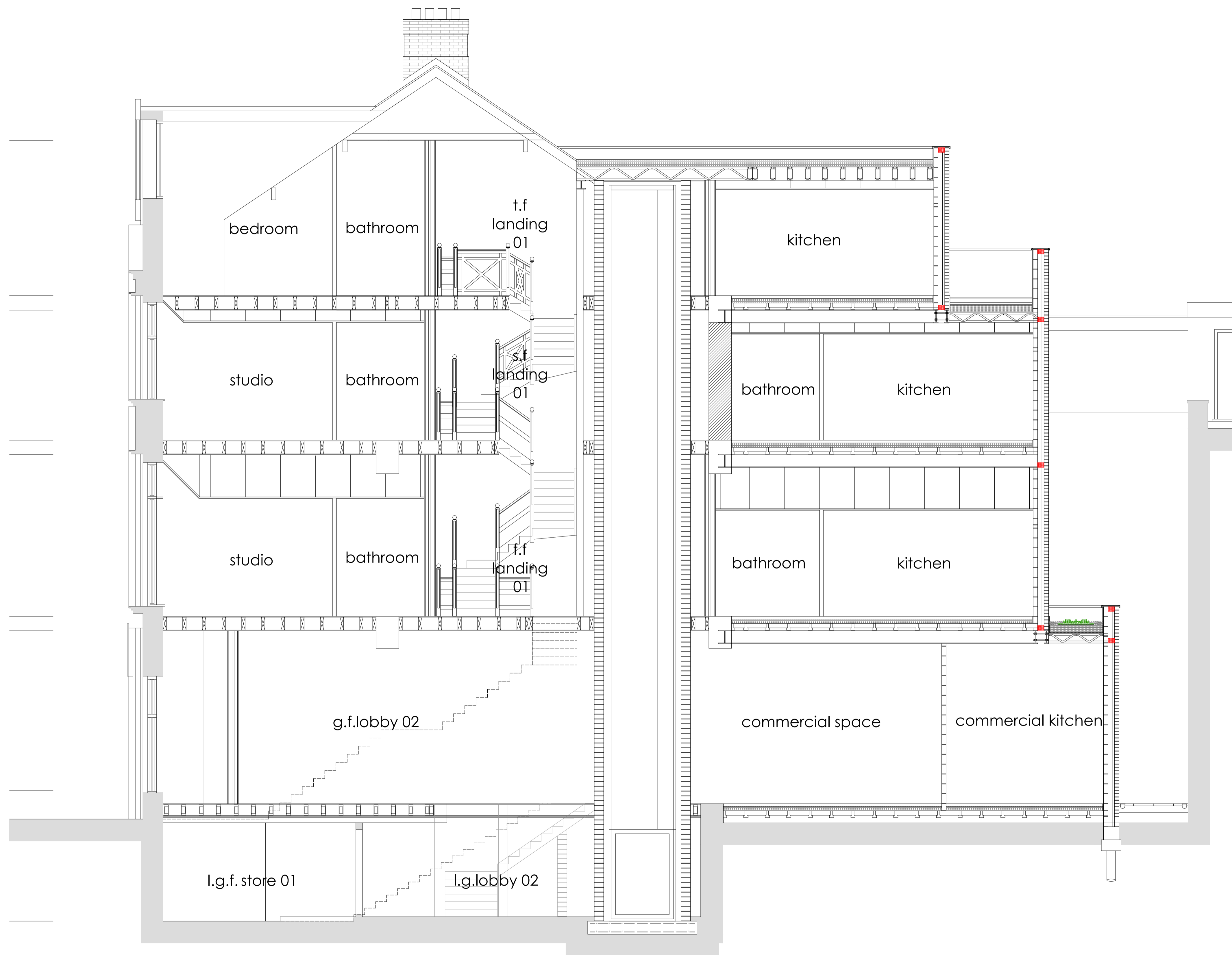
section a-a
